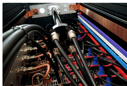
RED DE TOMA A TIERRA EN COBRE
