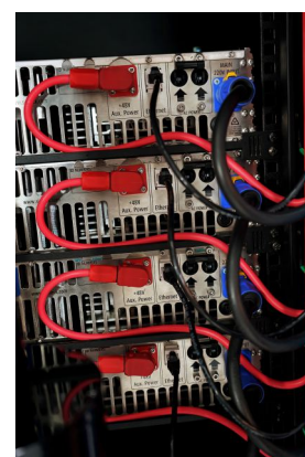
CONEXIÓN DC BLADES
